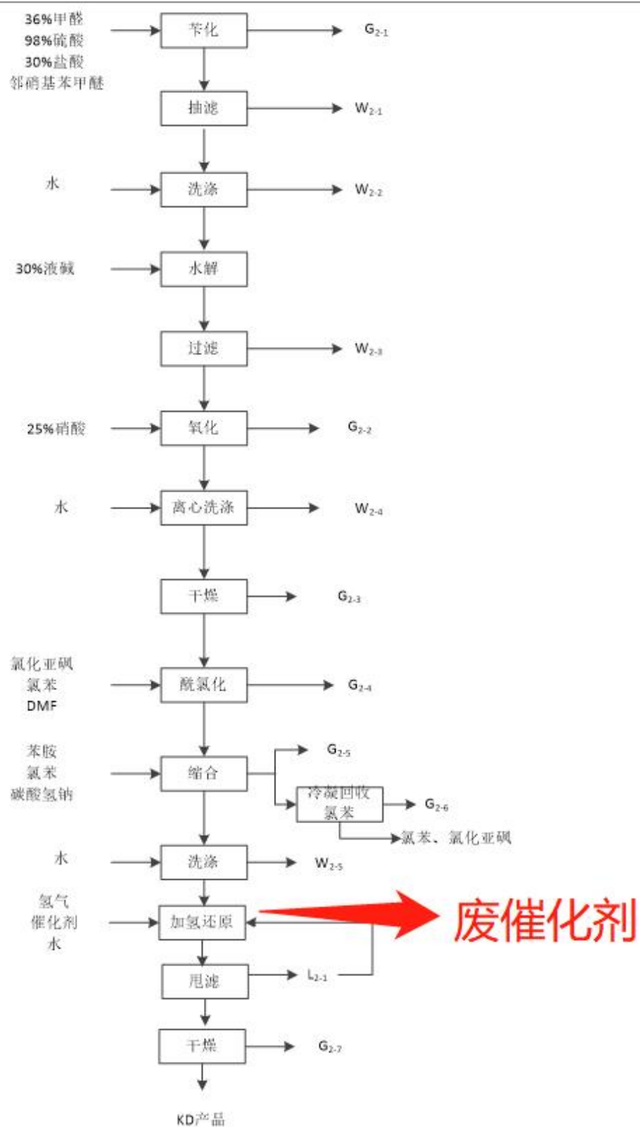
图3.4-1 技改后红色基KD生产工艺及产污环节示意图
